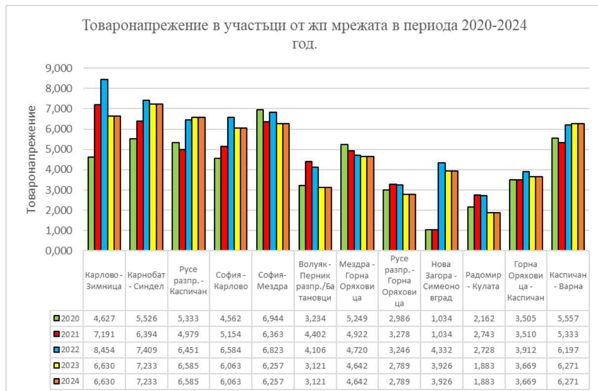
Графика № 11. Товаронапрежение по наблюдаваните жп линии за периода 2020-2024 г.
