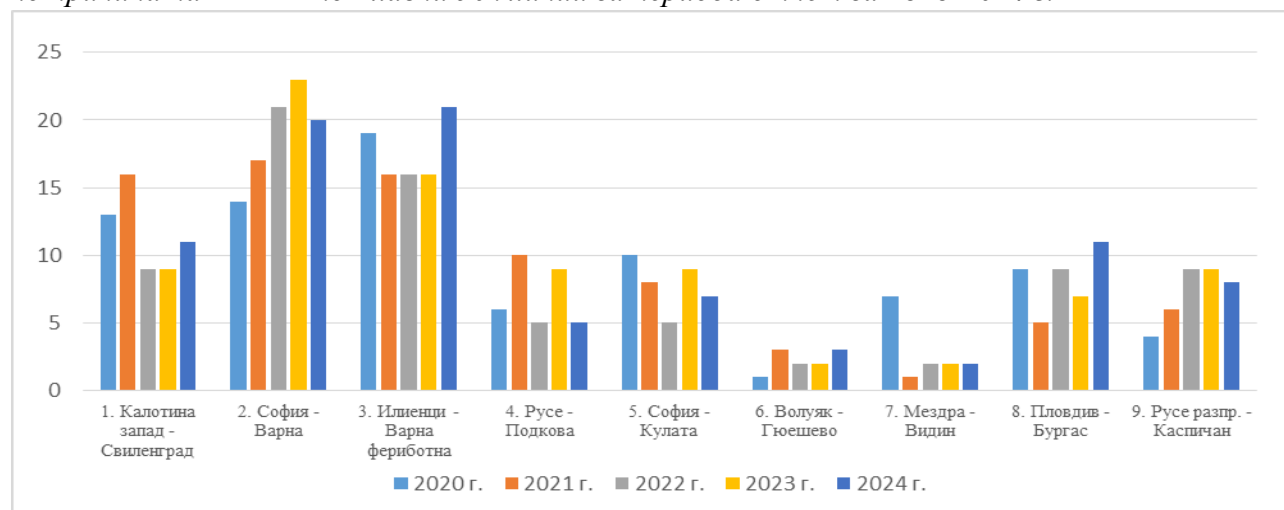
Графика № 17. Динамика на регистрираните събития по безопасността на превозите по причина на НКЖИ по Главни жп линии за периода отчет за 2020-2024 г.
